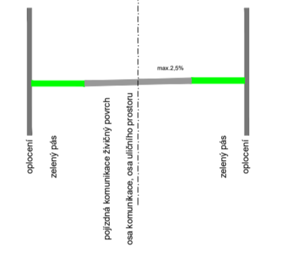
SCHÉMA PŘÍČNÉHO ŘEZU MOK 02 A 03
