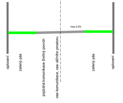
SCHÉMA PŘÍČNÉHO ŘEZU MOK 02 A 03
